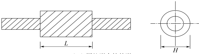
(b) 圆柱形套筒外形
