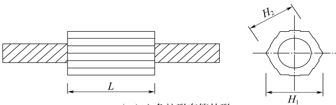
(a) 六角柱形套筒外形
